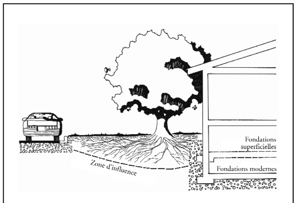
Figure 5 : Rapport entre un arbre à maturité et les fondations d'un bâtiment, là où l'arbre a été planté près du bâtiment.
