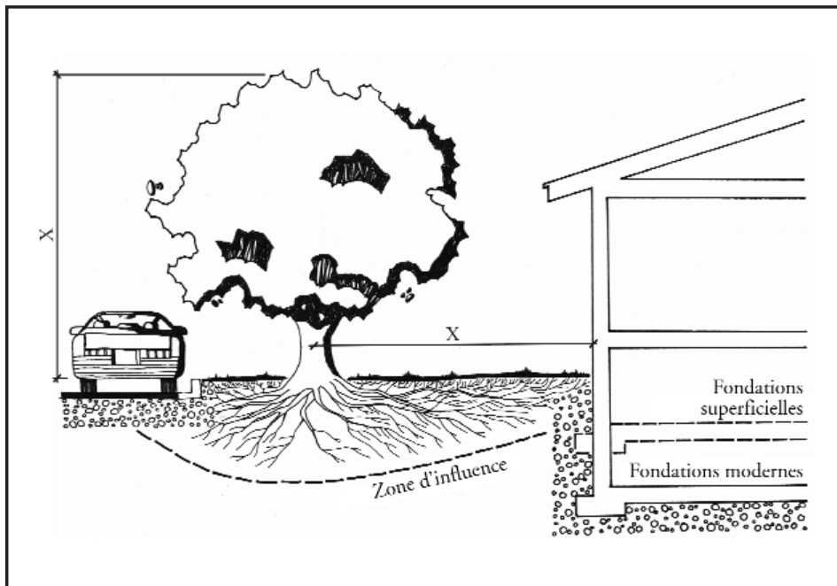
Figure 4 : Rapport entre un arbre à maturité et les fondations d'un bâtiment, là où la hauteur d'un arbre à maturité équivaut à la distance le séparant du bâtiment
